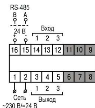
Рисунок 5.5 – Общая схема подключения ТРМ1–Щ5
