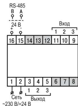
Рисунок 5.6 – Общая схема подключения ТРМ1–Д
